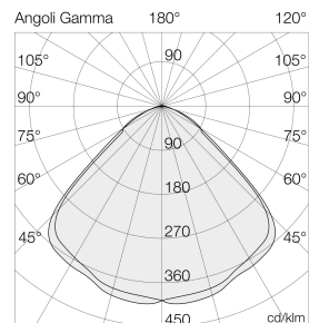
Ausleuchtung (Richtwert) 8400SU - Raum 8400SU4080 - 10000 lm Höhenleiter 40° (90° - 140°) 100° (200°)
