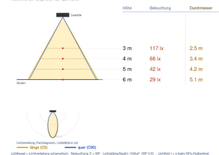
Ausleuchtung (Richtwert) 8401CU4080GL - 80W 4000K Silber Höhenabstand 20° (10° / 30°) 100° (10° / 30°)
