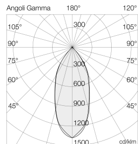
Ausleuchtung (Richtwert) 8401CU4170GL - Raum 8401CU4170GL - 20000 lm Höhenwerte 20° (3m) - 10° (4m) - 5° (5m) - 3° (6m)
