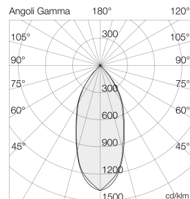
Ausleuchtung (Richtwert) 8401CU4190GL - Raum 8401CU4190GL - 20000 lm Höhenleiter 20' (6,1m) - 100' (30,5m)
