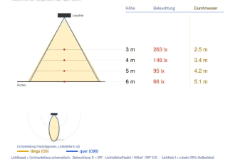
Ausleuchtung (Richtwert) 8401CU4190GL - Raum 8401CU4190GL - 20000 lm Höhenleiter 20' (6,1m) - 100' (30,5m)
