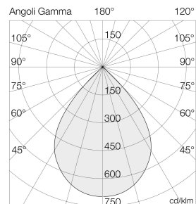
Ausleuchtung (Richtwert) 8401S2 - max 8401S24120 - 1.0000 lx Höhenwert 27° (100°) - 20° (100°)
