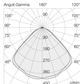
Ausleuchtung (Richtwert) 8401SU - 80W 4000K 1000mm Höhenbereich 40° (SU) - 40° (SU)
