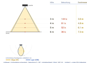
Ausleuchtung (Richtwert) 8402S24280GL (S2) 280W 4000K Silber Halbwinkel (°) / Höhe (m) / Durchmesser (m)
