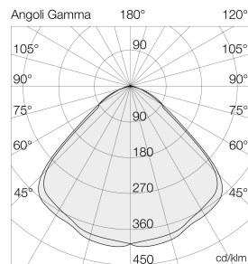
Ausleuchtung (Richtwert) 8402SU - 180° 4000K/200W Höhenwerte 40° (30°) 40° (30°)
