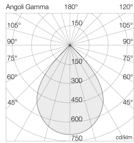
Ausleuchtung (Richtwert) 8407S24130GD - 130W/4000K/500lm - 1200mm H Halbkegel 31° (Ang. 0.5) - 20° quer (0.5)
