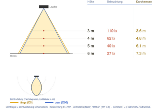
Ausleuchtung (Richtwert) 8407S24130GD - 130W/4000K/500lm - 1200mm H Halbkegel 31° (Ang. 0.5) - 20° quer (0.5)
