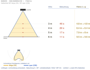
Ausleuchtung (Richtwert)
