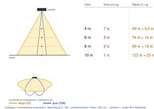
Ausleuchtung (Richtwert) 9202CP - MIG 1B (CP) 50W 4000K CRI 70 Silber Halbwinkel 81° (81°/105°) 40° (40°/55°) asymmetrisch CP40
