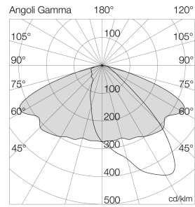
Ausleuchtung (Richtwert) 9202ME - 1x 75W 3000K (E17) - 11000 lm Halbwertsbreite 51° (typ.) / 10° (max.) - asymmetrische Optik
