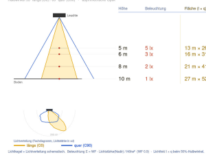
Ausleuchtung (Richtwert)
