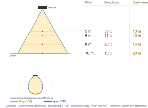
Ausleuchtung (Richtwert) 9300RA4054RD - 54W 4000K Grafite - 10000 lm Halbwinkel 40° (Ang. 105° - 40° quer (20°))
