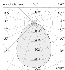
Ausleuchtung (Richtwert) 9300RA4054RD - 54W 4000K Grafite - 10000 lm Halbwinkel 40° (Ang. 105° - 40° quer (20°))
