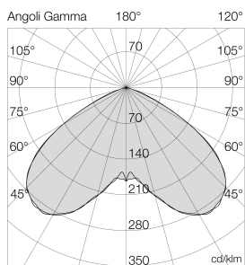
Ausleuchtung (Richtwert) 9302/RT - HAN 9302/RT4015 | 2498 lm Halbwinkel 61° längs (C0) / 59° quer (C90)
