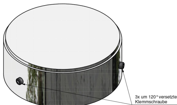
Stahlkappe für Zopf-Ø 133 - 139
