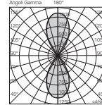
mod.B6 Biemissione 60°
