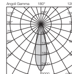
mod.M3 Spot 36°
